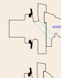
Profil traverse intermédiaire à bec de corbin
